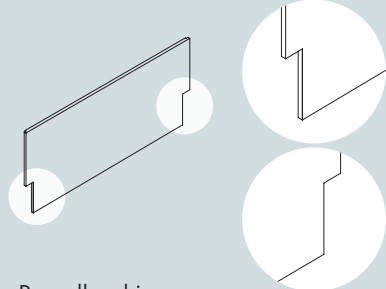
Pannello schiena con scasso sinistro e destro Right and left shaped back panel
