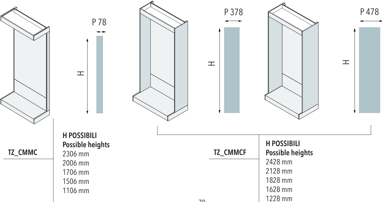
COPRIMONTANTE CON BASE E CON CELINO Cover for wall upright with base and with canopy
