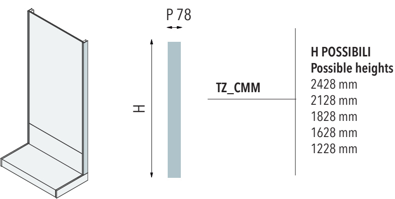
COPRIMONTANTE CON BASE NO CELINO Cover for wall upright with base no canopy
